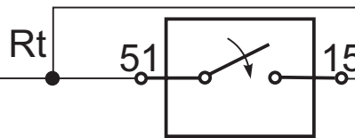
Zündschloß (ignition lock)
